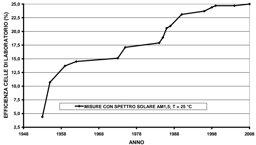
Fig.2 – Serie storica dell'efficienza di conversione delle celle al silicio monocristallino in versione da laboratorio d'area pari a 4 \text{ cm}^2 . Fonti: archivio storico dell'autore e "Solar Cell Efficiency Tables, (Green et al., 2009)
