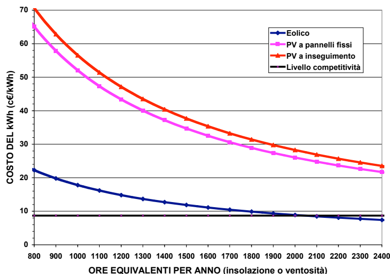
Fig.2 - Costo del kWh per eolico e fotovoltaico in funzione della produttività energetica potenziale del sito. Il livello di competitività è posto a 8,7 c€/kWh secondo il valore medio del 2008 fissato per il prezzo unico dalla AEEG nel Rapporto Annuale di Attività 2009.
