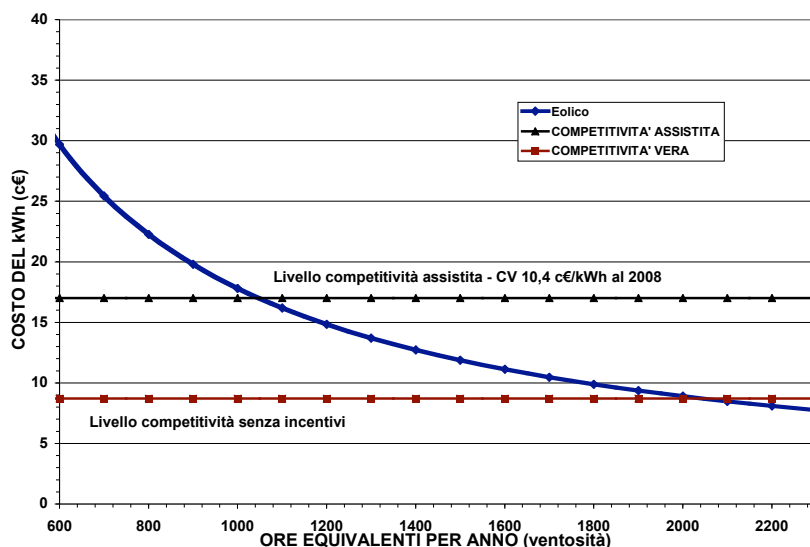
Fig.3 - Costo del kWh eolico a confronto con il livello di competitività assistita posto a 17 c€. Il costo scende sotto al livello di competitività a partire da 1050 ore equivalenti.
