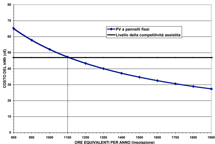
Fig.5 - Costo del kWh per impianti fotovoltaici di piccola taglia a pannelli fissi con il livello di competitività assistita posto a 47,0 c€. Il costo scende sotto al livello di competitività a partire da 1100 ore equivalenti.
